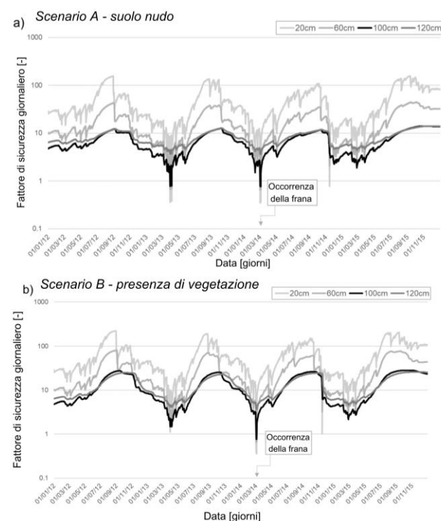
Fig.3 – Risultati per il calcolo del fattore di sicurezza giornaliero per due scenari distinti: A) suolo nudo; B) presenza di vegetazione.
