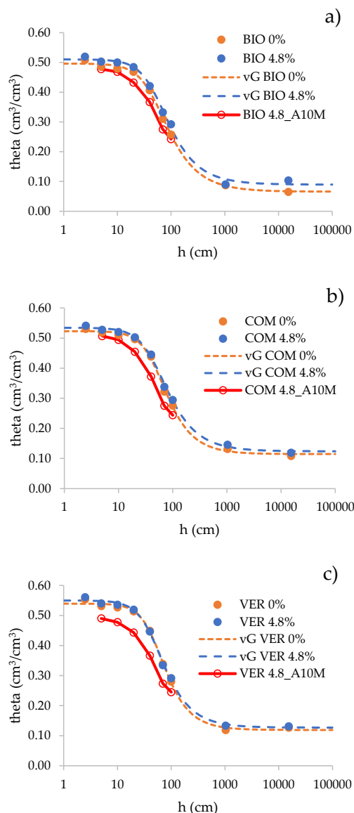
Fig.2 - Curve di ritenzione idrica corrispondenti all'ammendamento del suolo con biochar (a), compost (b) e vermicompost (c), alle due concentrazioni (0 e 4.8%). In tratteggio sono state riportate le curve interpolanti le misure sperimentali ottenute con il modello vG. Le misure ripetute dopo 10 mesi (A10M) sono evidenziate in rosso.
